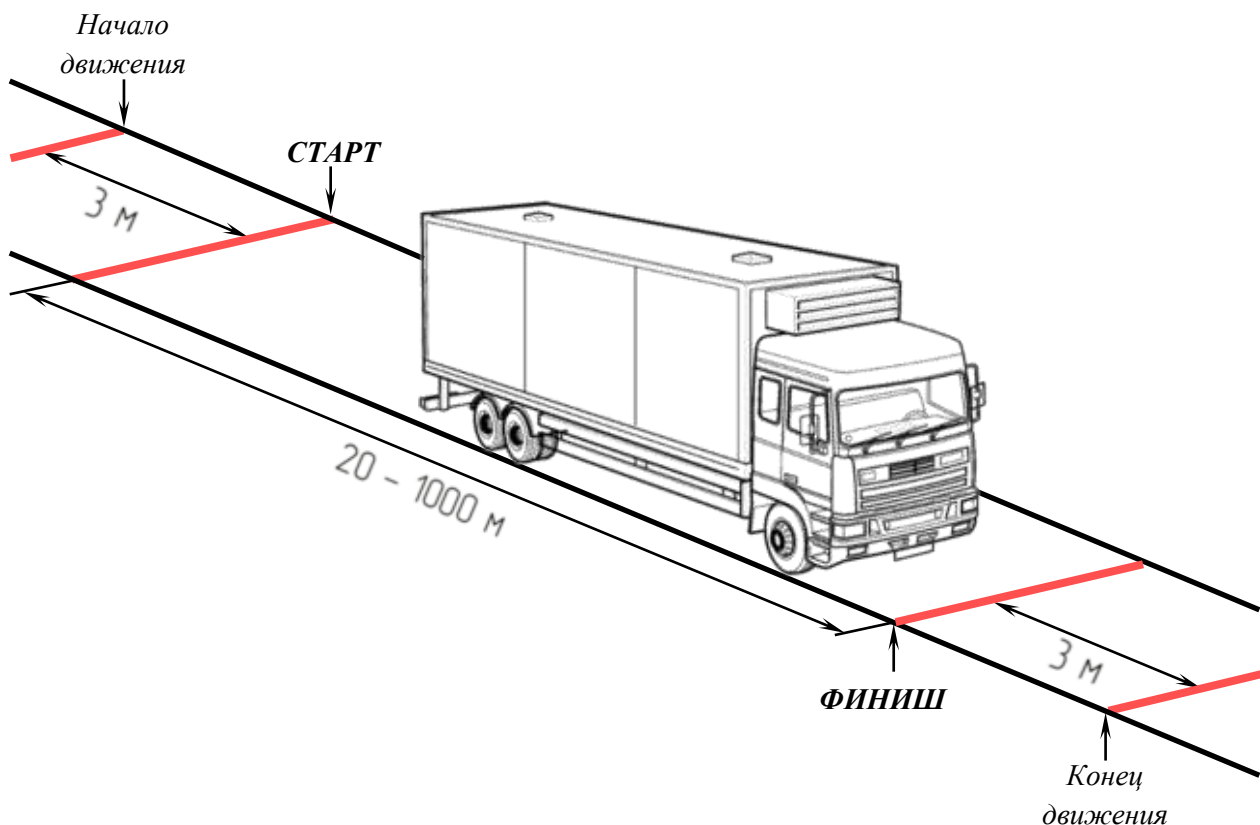
Рисунок 21. Определение параметра w прокаткой по тестовой площадке
