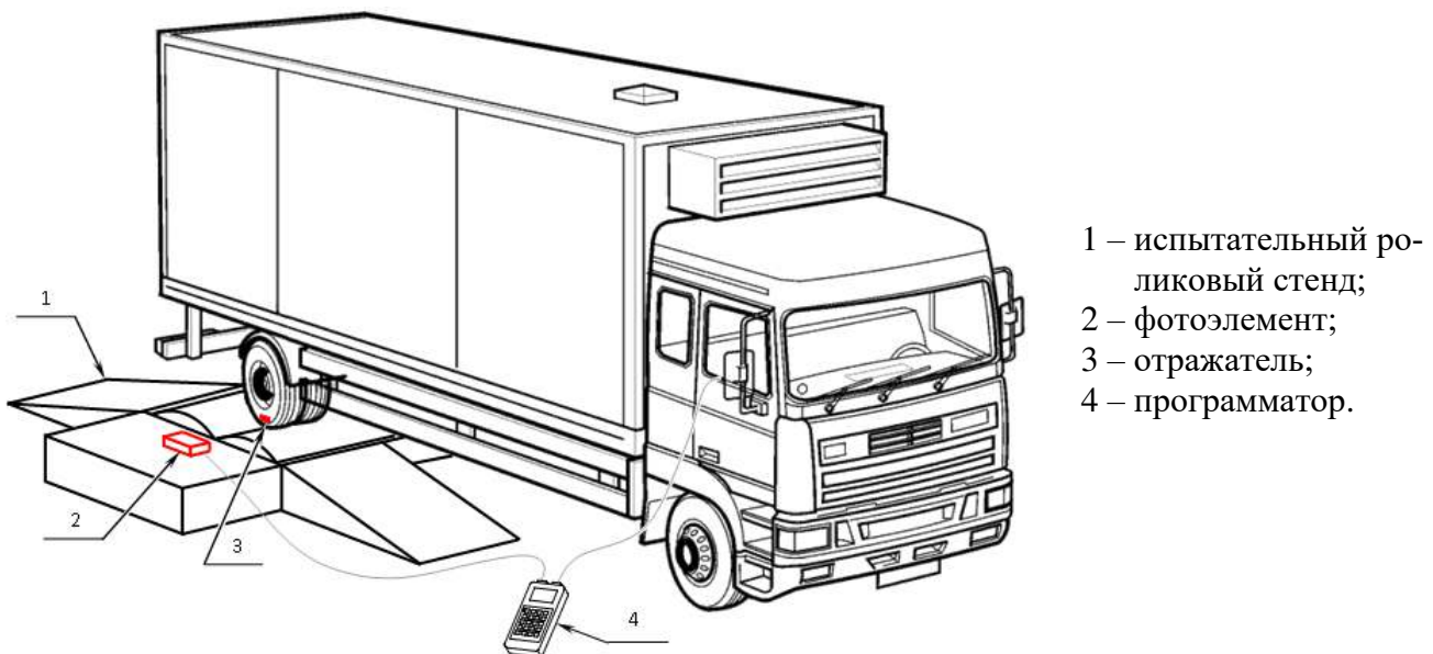
Рисунок 22. Определение параметра w на роликовом стенде
