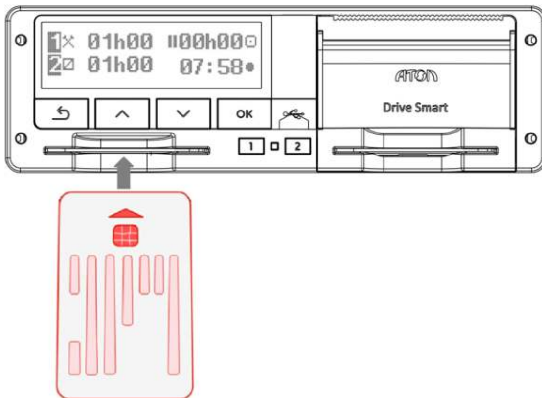
Рисунок 16. Установка карты
