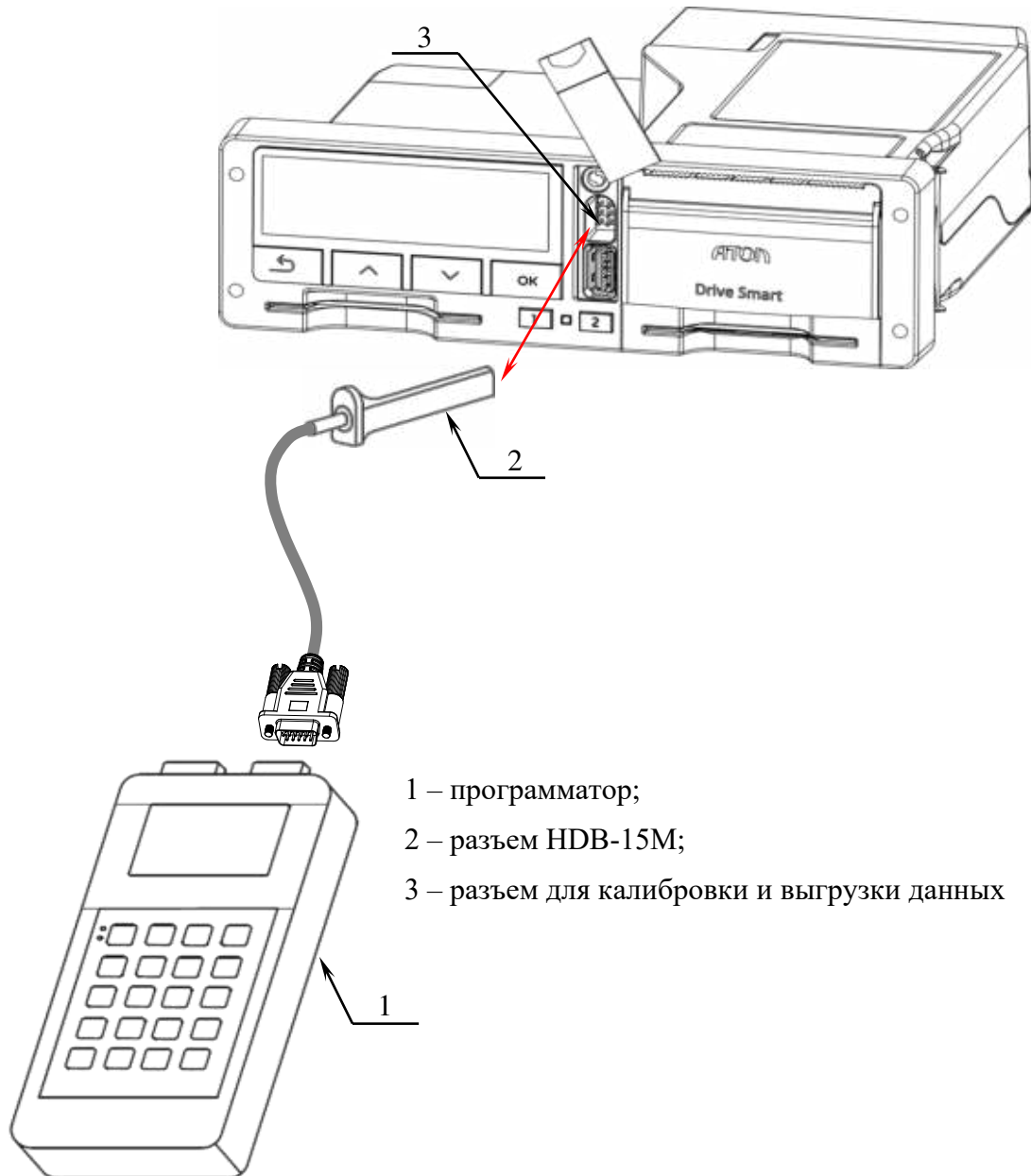
Рисунок 23. Подключение программатора
